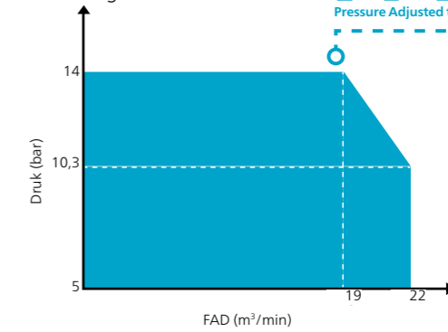
Prestatiegrafiek: XAVS 378
