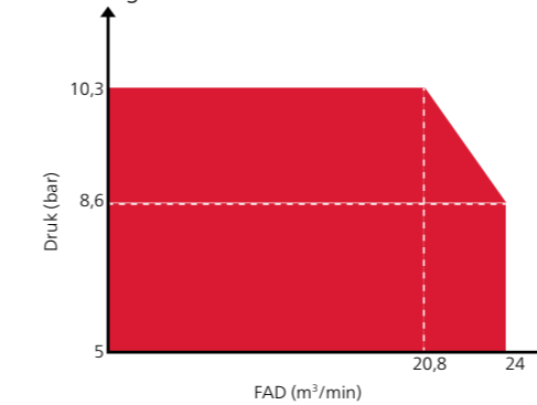
Prestatiegrafiek: XAHS 408
